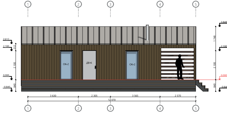
Фасад в осях 1-5
