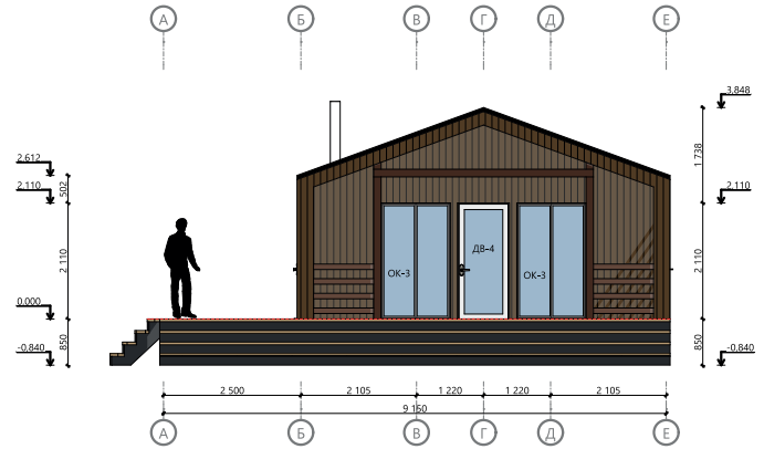
Фасад в осях А-Е
