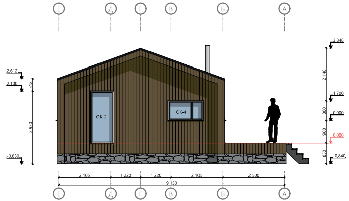
Фасад в осях Е-А
